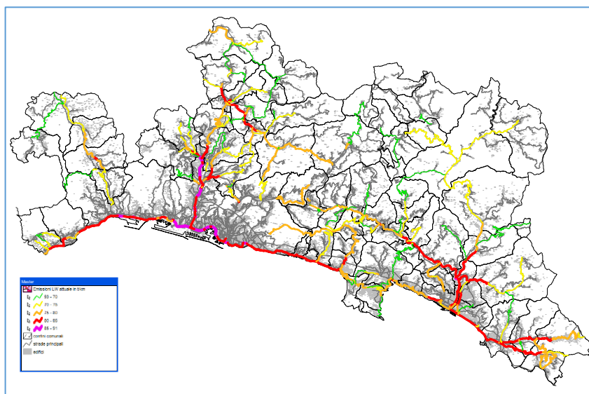
Livello di potenza sonora lineare medio pesato A della rete stradale provinciale riferito al periodo diurno (fonte PTVE, 2008).
